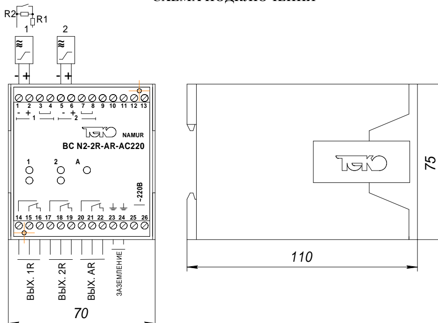
ГАБАРИТНЫЙ ЧЕРТЕЖ СХЕМА ПОДКЛЮЧЕНИЯ
